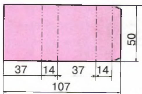
1 коробка
